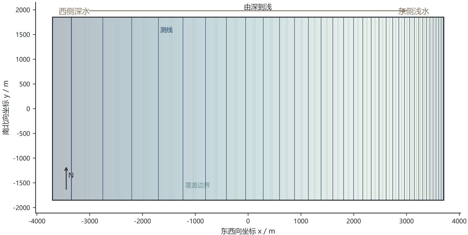
规则坡面测线布设与覆盖条带
