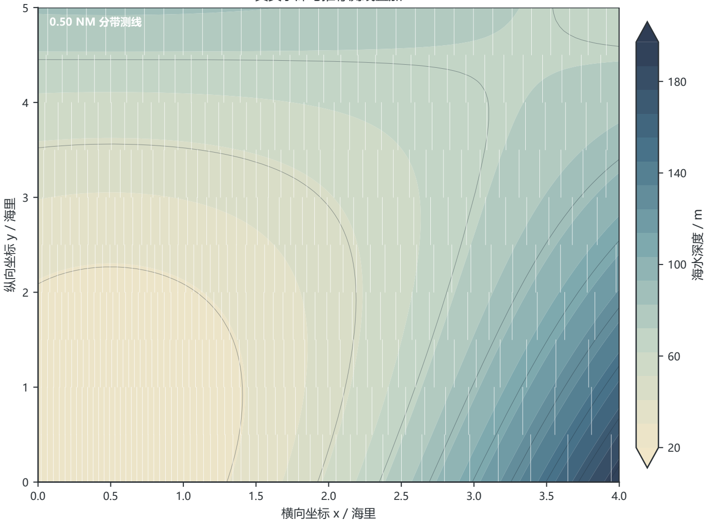
真实水深与推荐测线叠加
