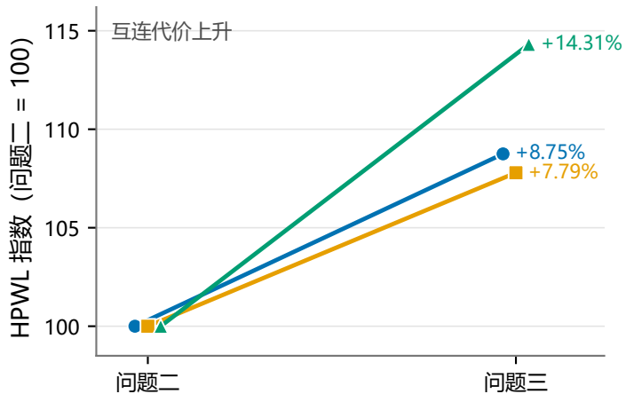
(b) HPWL 代价
