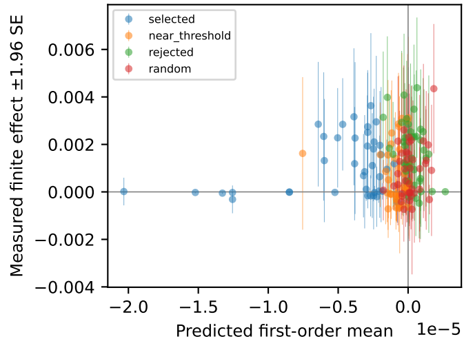
llama8b N16 CE
