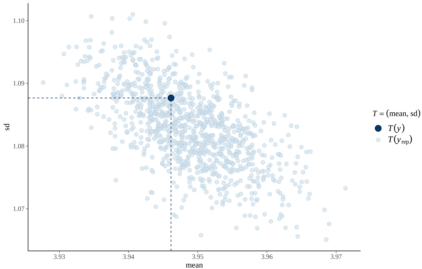
Posterior predictive check (2d stat)
