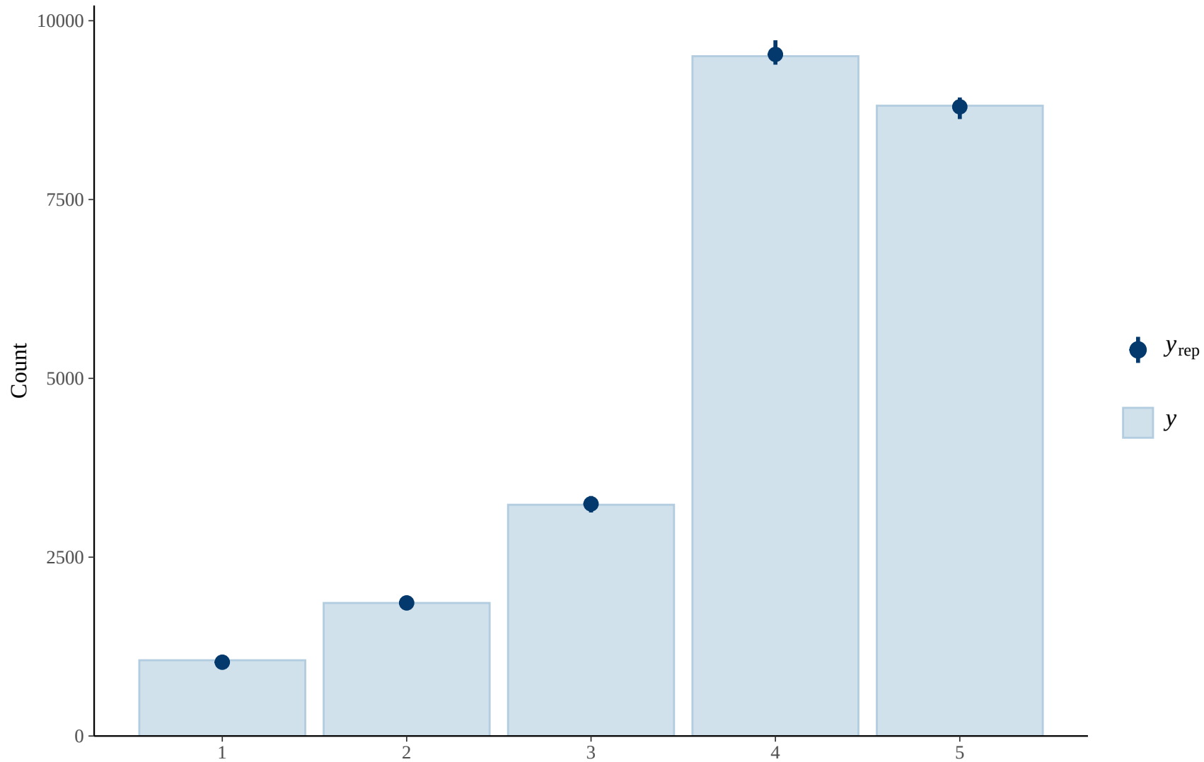
Posterior predictive check (bars)
