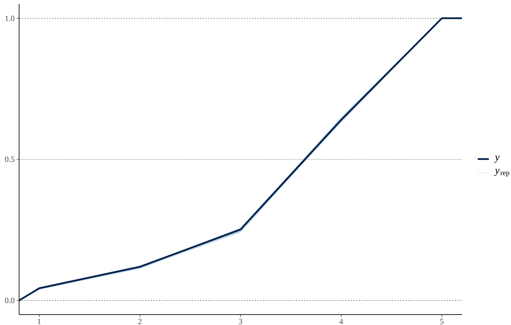
Posterior predictive check (ECDF)
