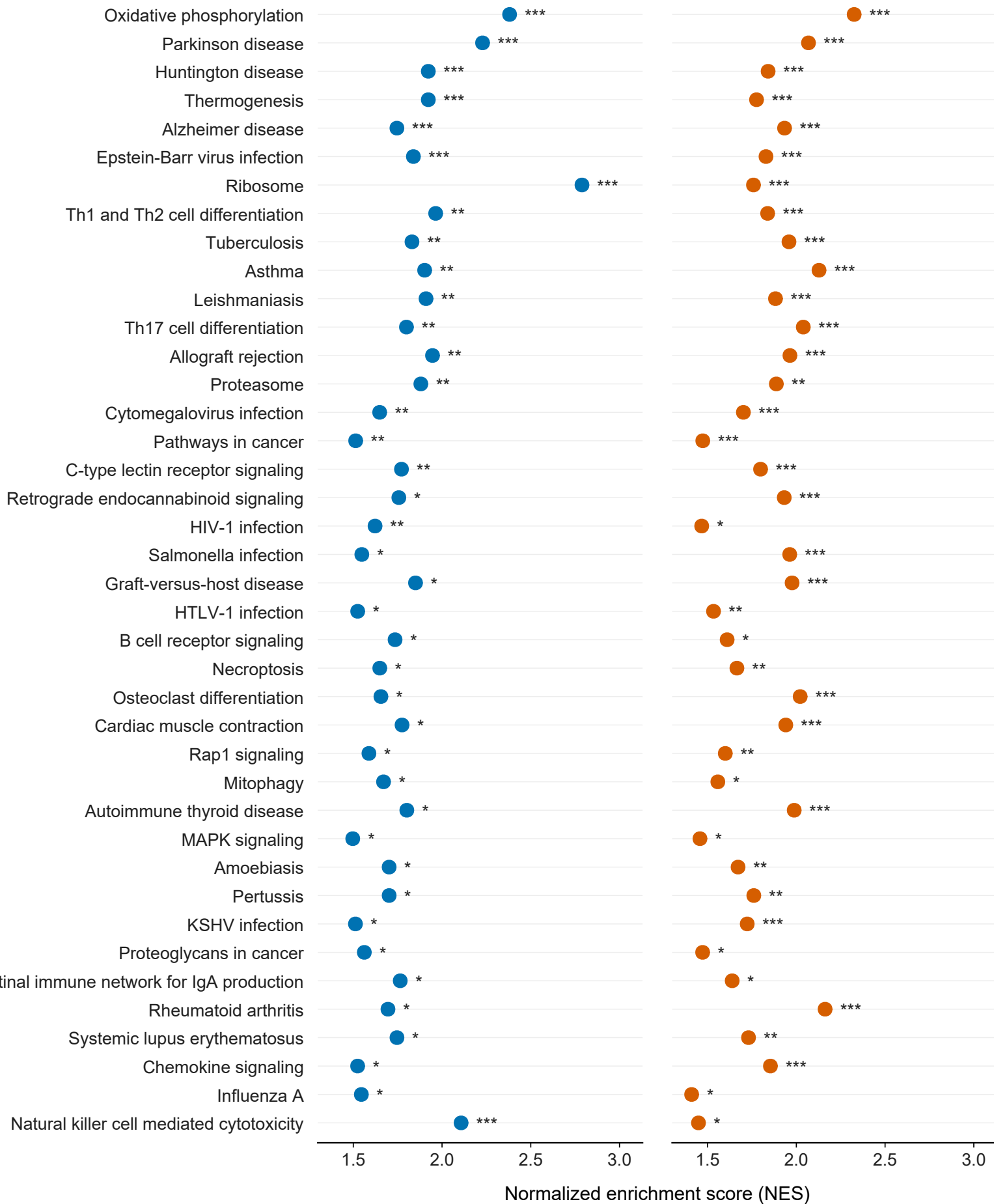
Relapse scRNA-seq
