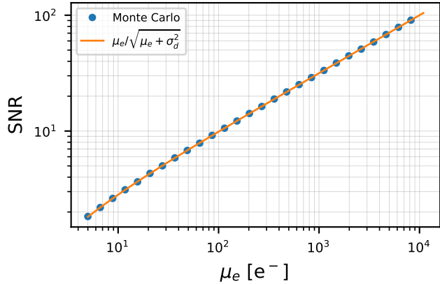
Temporal SNR
