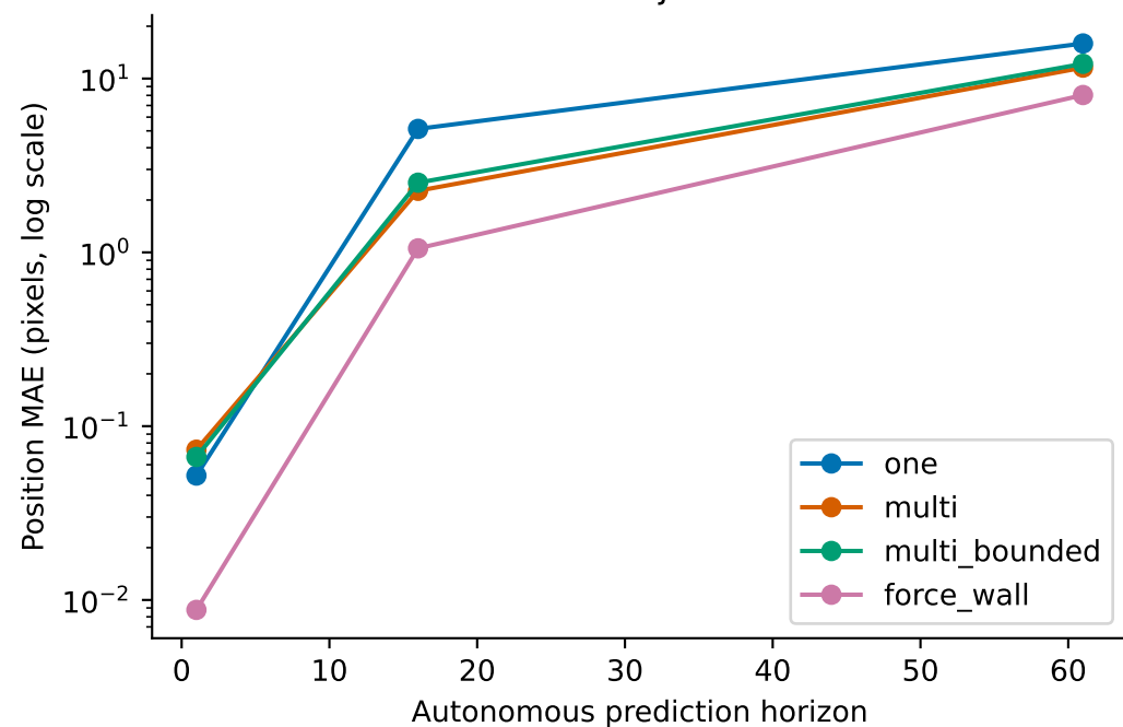
oracle
