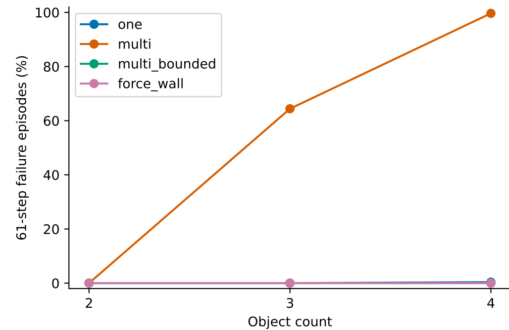
oracle
