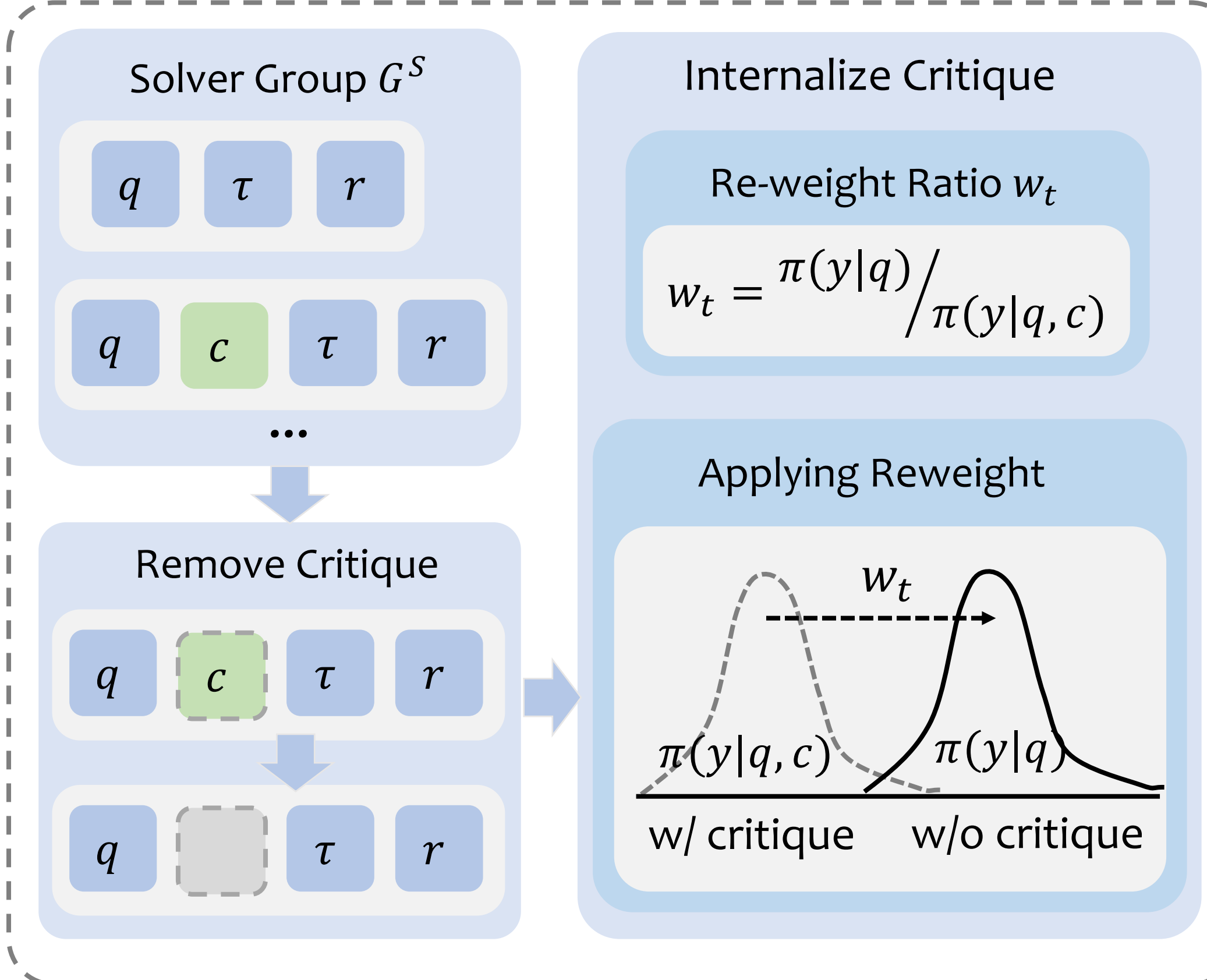
(b) Internalize Critique
