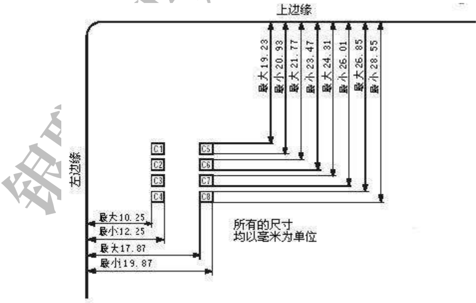
图 20 银联标识下置格式时的芯片卡规格示意图
