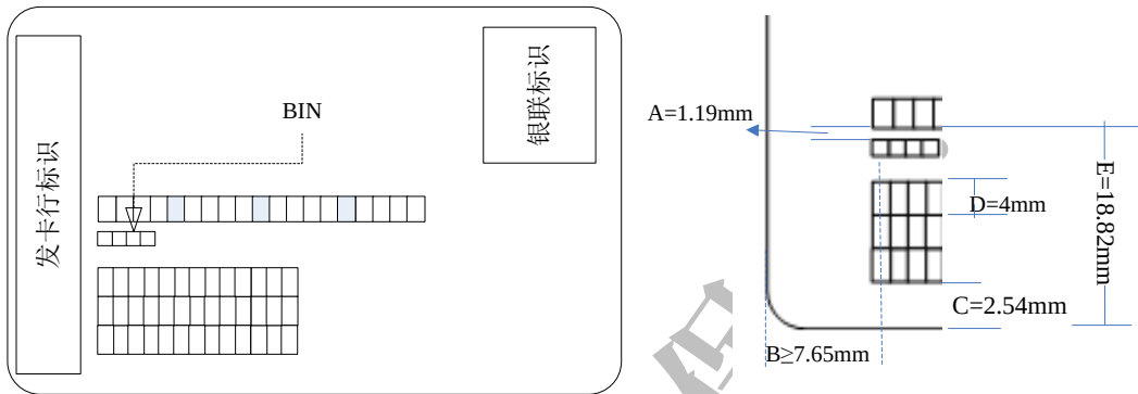
图30 版式二凸印/平印区规格
