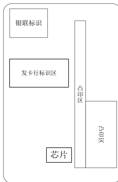
图32 版式二中接触式芯片的位置
