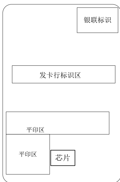
图31 版式一中接触式芯片的位置
