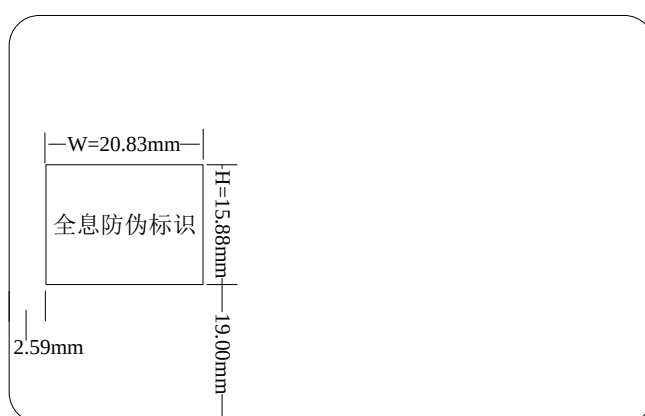
图36 全息防伪标志在卡片上的位置
