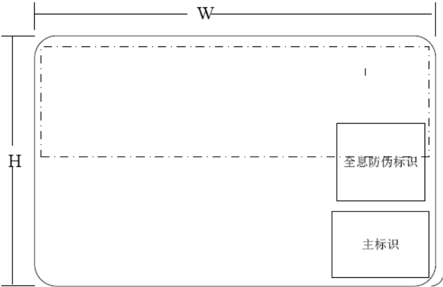
图 1 银联卡卡片外形 表 1 银联卡标准卡片尺寸
