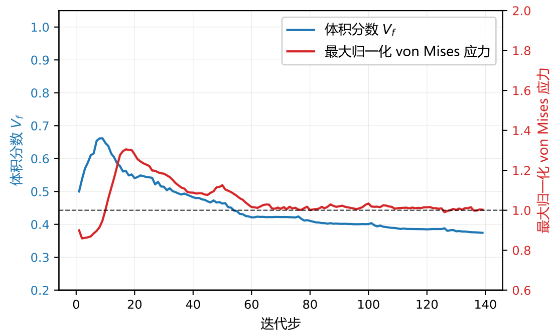
(c) 胡张混合法 ( k=2 ) 收敛历史
