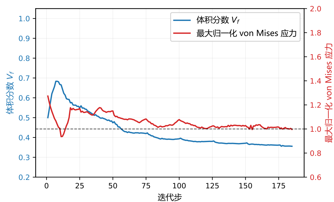
(a) 标准位移法 ( k=2 ) 收敛历史
