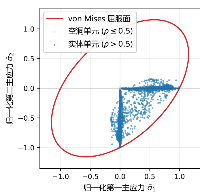
(b) 标准位移法 ( k=2 ) 主应力分布
