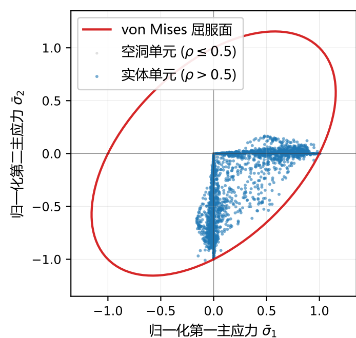
(d) 胡张混合法 ( k=2 ) 主应力分布
