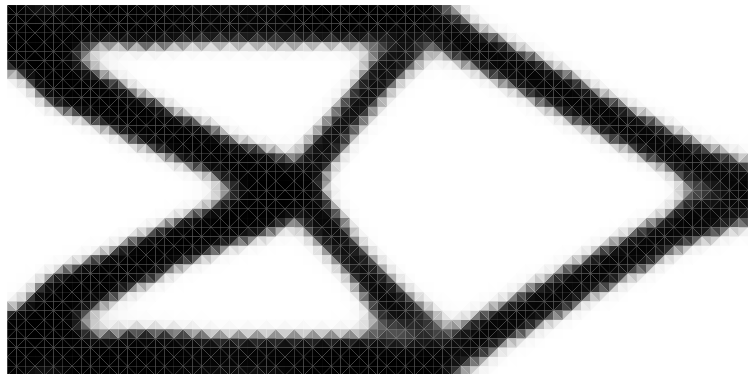
(c) 胡张混合法 ( k = 4 ) 最终拓扑构型 ( V^* = 36.06\% )
