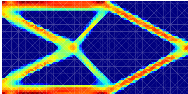
(d) 胡张混合法 ( k = 4 ) 归一化 von Mises 应力
