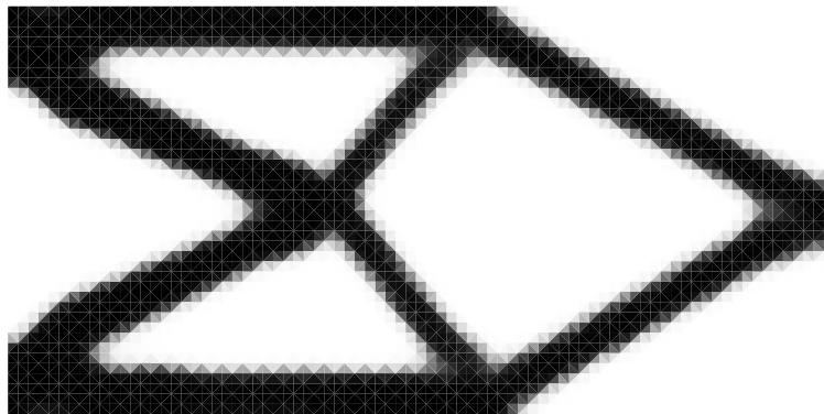
(a) 胡张混合法 ( k = 3 ) 最终拓扑构型 ( V^* = 35.51\% )
