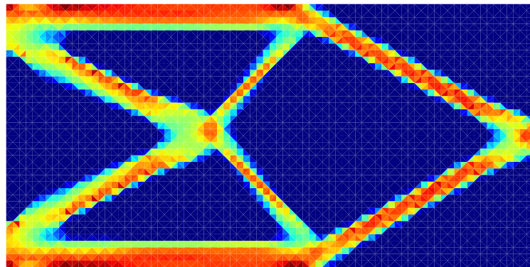
(b) 胡张混合法 ( k = 3 ) 归一化 von Mises 应力
