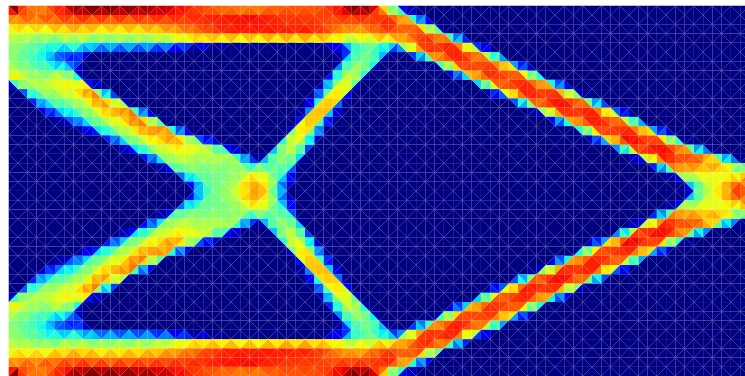
(b) 标准位移法 ( k = 2 ) 归一化 von Mises 应力
