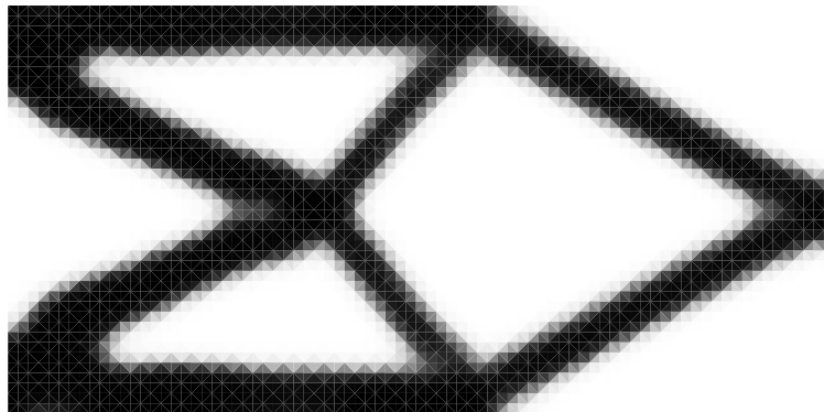
(c) 胡张混合法 ( k = 2 ) 最终拓扑构型 ( V^* = 37.39\% )
