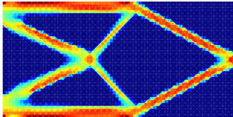
(d) 胡张混合法 ( k = 2 ) 归一化 von Mises 应力
