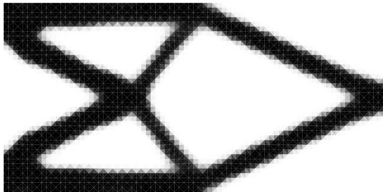
(a) 标准位移法 ( k = 2 ) 最终拓扑构型 ( V^* = 35.55\% )
