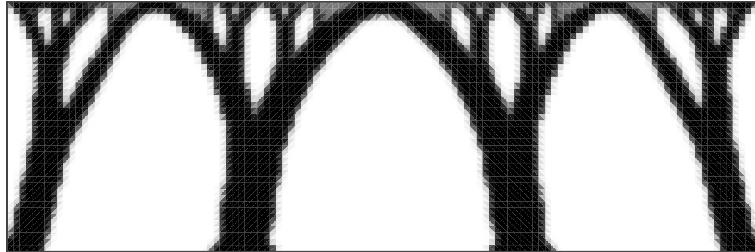
(d) LFEM ( p = 2 , \nu_0 = 0.4999 , C = 98.06 )
