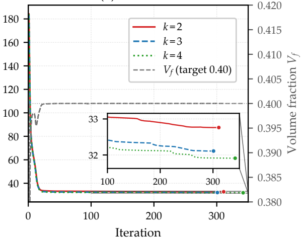
(b) HZMFEM
