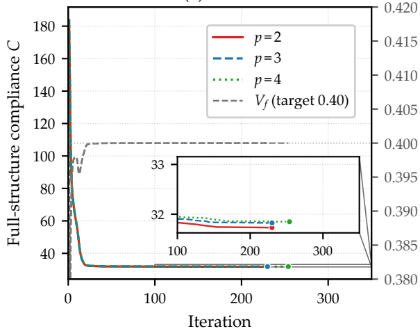
(a) LFEM
