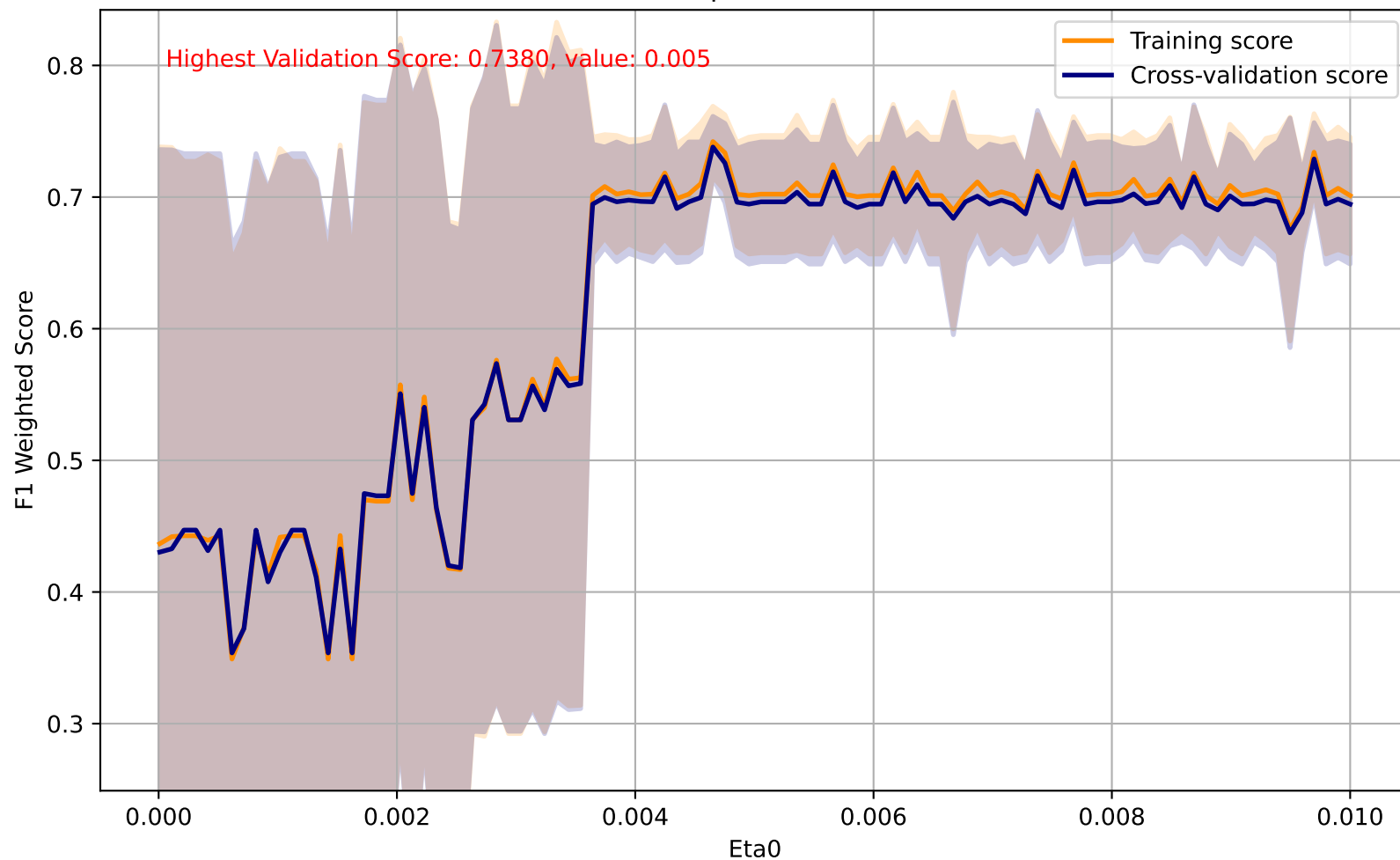
Perceptron - Eta0
