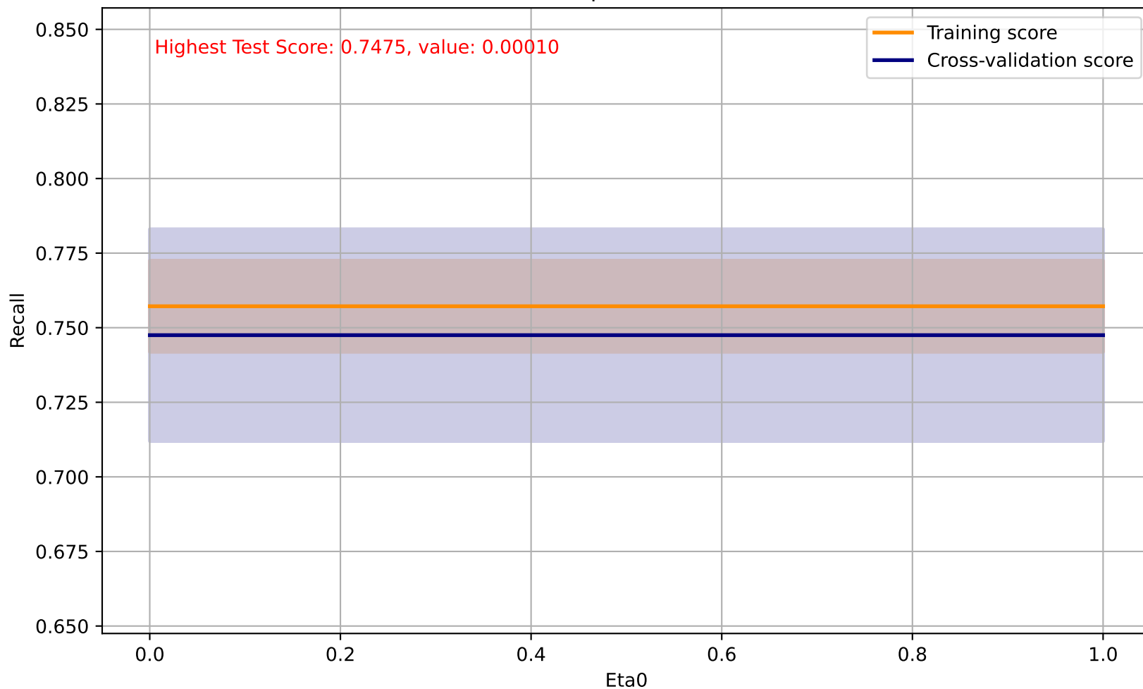
Perceptron - Eta0
