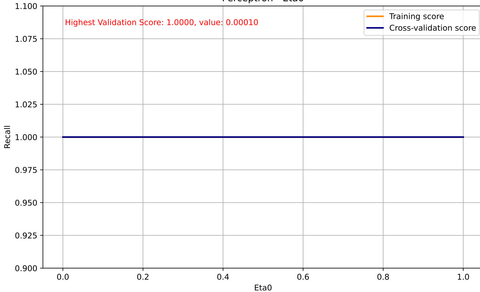
Perceptron - Eta0
