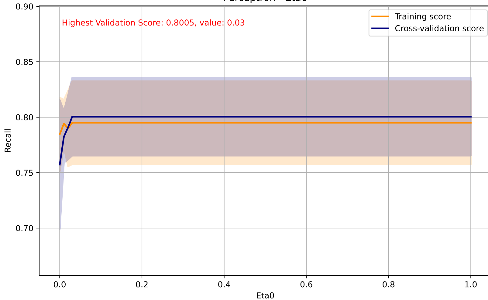
Perceptron - Eta0
