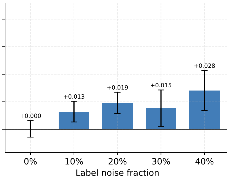
CUB-200
