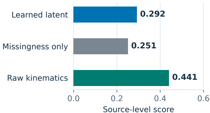
Macro-F1
