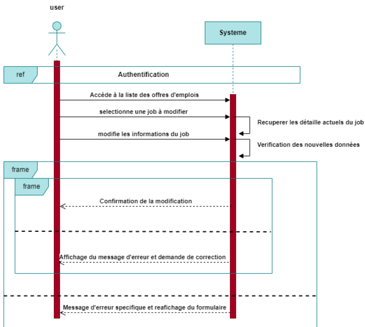
Figure 8 : Diagramme de séquence modification d'une offre
