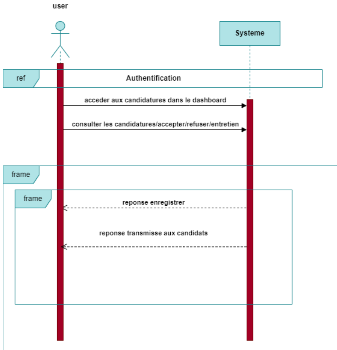
Figure 10 : Diagramme de séquence consultation des candidatures
