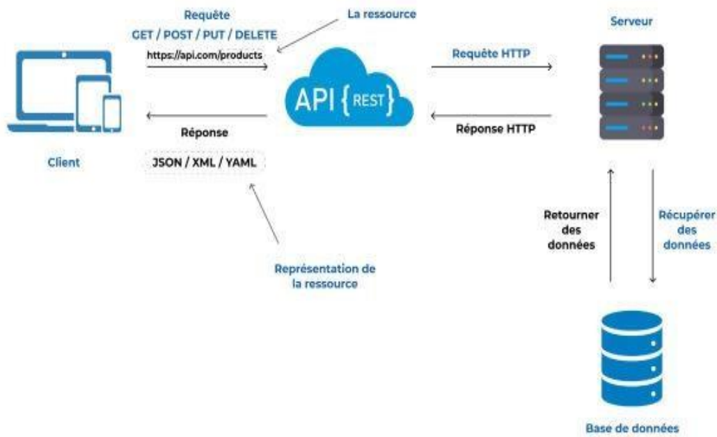
Figure 3 : Architecture du système
