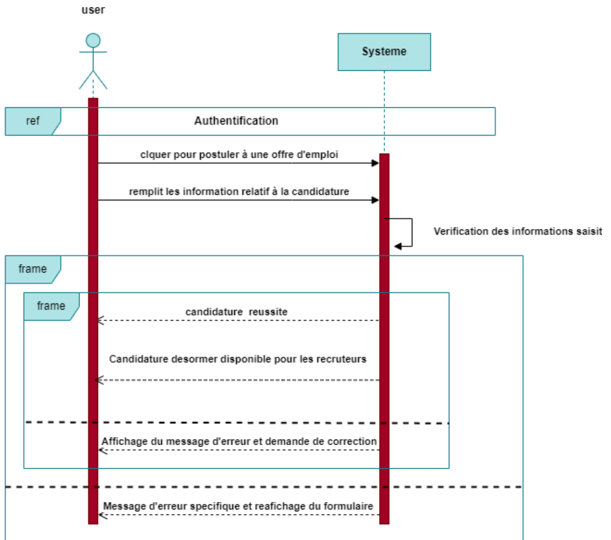
Figure 9 : Diagramme de séquence pour postuler
