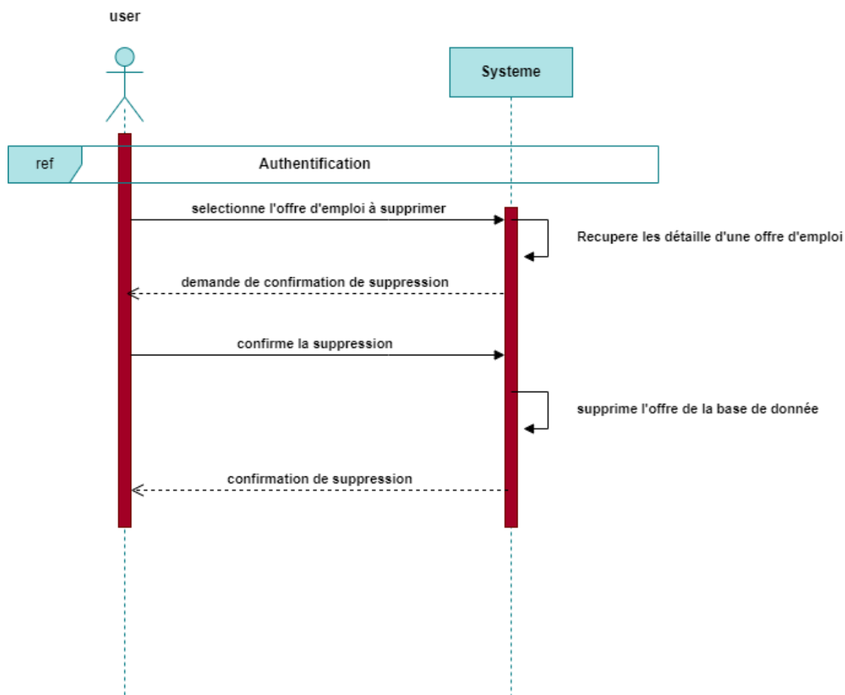
Figure 11 : Diagramme de séquence suppression d'une offre
