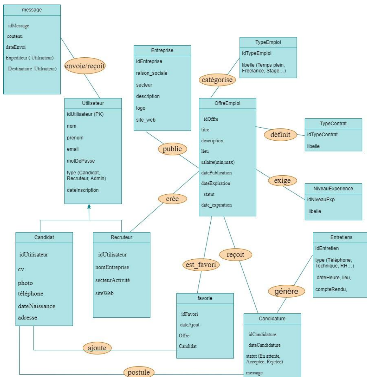
Figure 12 : Modèle Conceptuel de données
