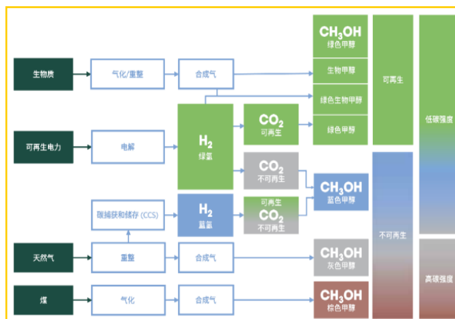
图表31: 甲醇制取技术路线图
