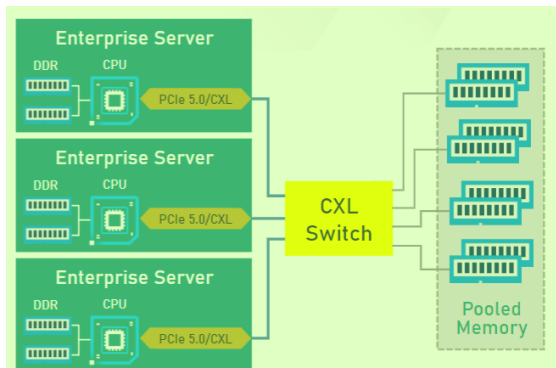
图35 CXL 2.0 机架级内存池化 2
