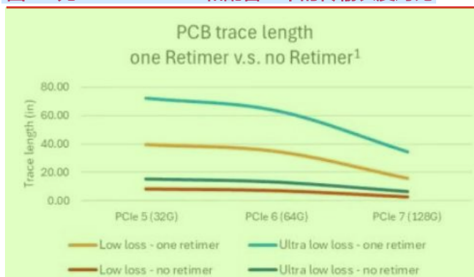
图28 无 PCIe Retimer 和配备一个的传输长度对比 6
