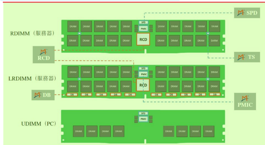
图25 公司内存模组配套芯片在典型内存模组中的位置分布 5
