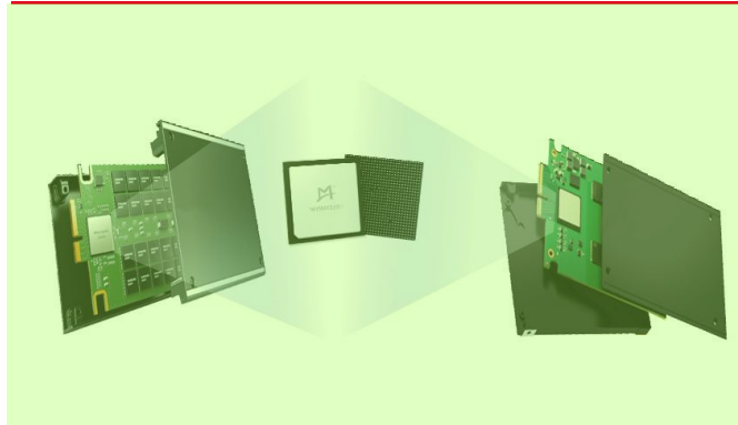
图39 CXL MXC 芯片在 EDSFF 内存模组中的产品应用形态
