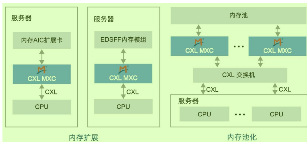
图37 CXL MXC 和 CXL Switch 典型应用场景 11
