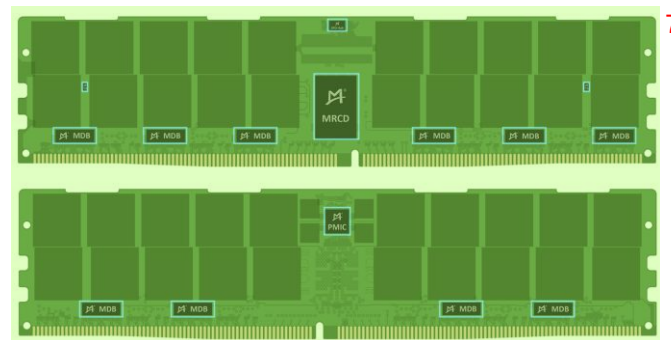
图12 DDR5 MRDIMM / MCRDIMM 内存接口芯片 6
