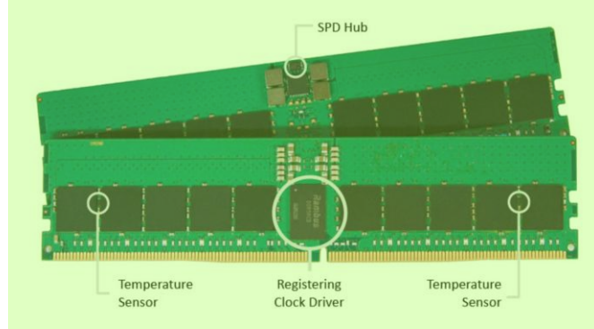
图21 Rambus DDR5 RDIMM 内存接口芯片 8
