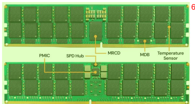
图20 瑞萨电子服务器 DDR5 MRDIMM 解决方案 5
