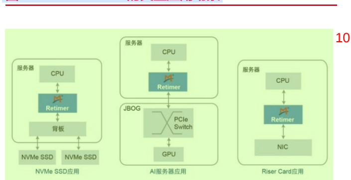
图29 PCIe Retimer 的典型应用场景 9
