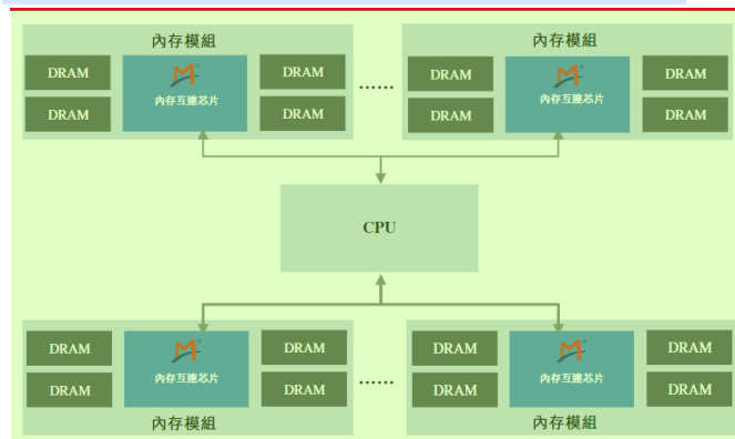
图11 计算机系统内存互连芯片与其他组件连接方式 3
