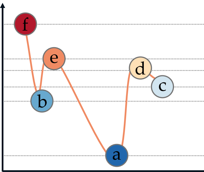
Scalar Function
