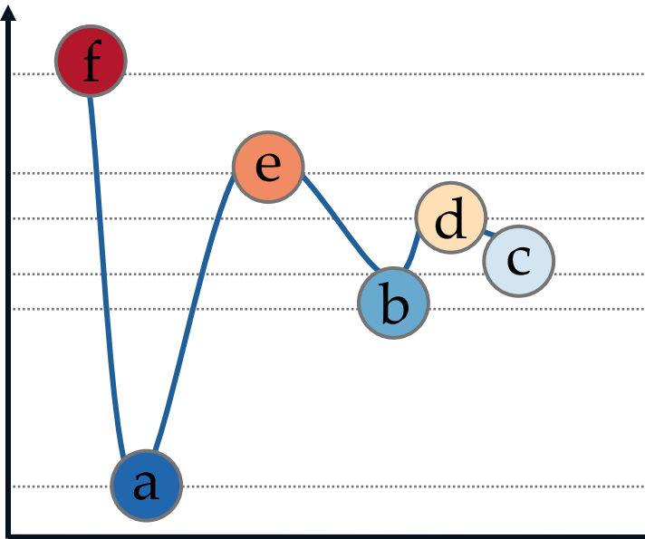
Scalar Function
