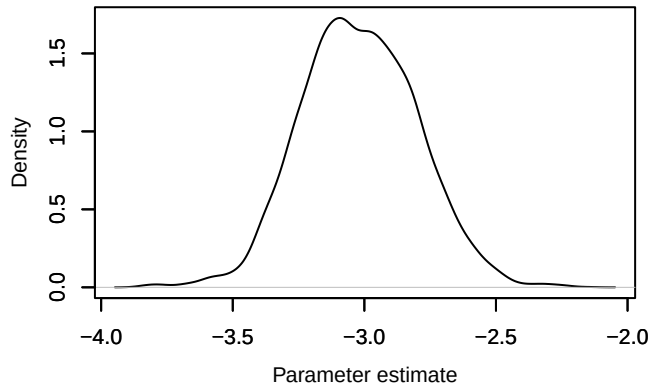
Density – b_post[1, 1]
