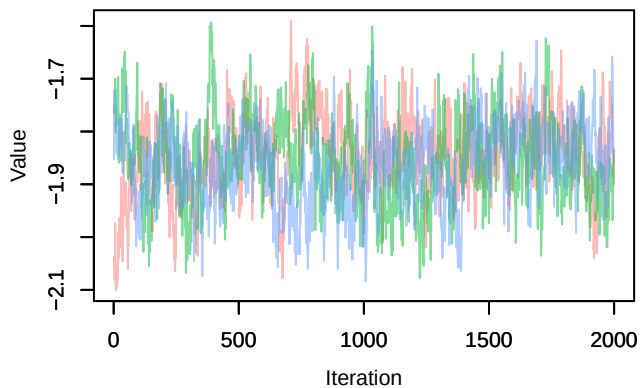
Trace – b_post[1, 2]
