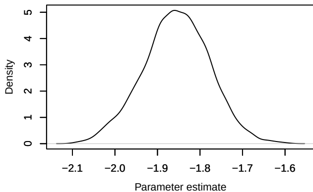
Density – b_post[1, 2]
