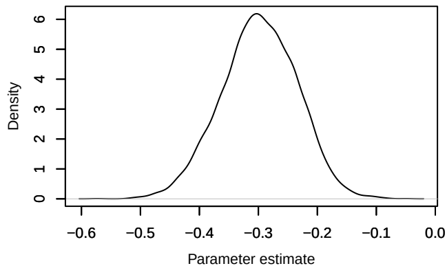
Density – b_post[1, 3]
