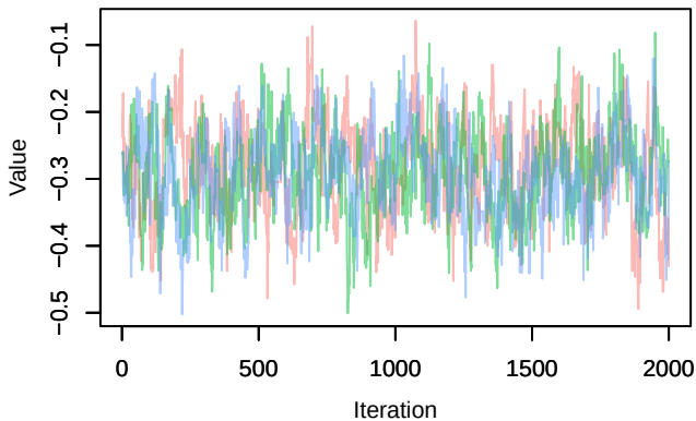
Trace – b_post[1, 3]
