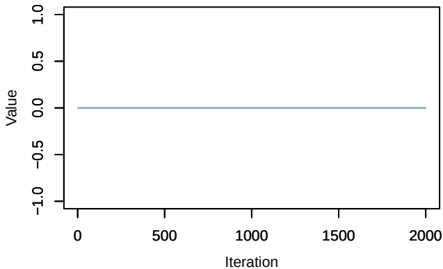
Trace – b_post[2, 3]
