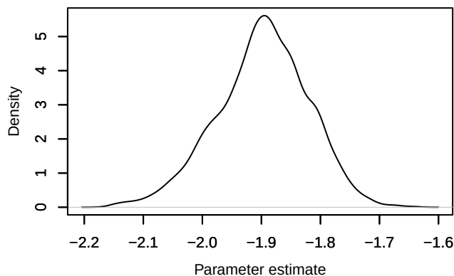
Density – b_post[1, 2]
