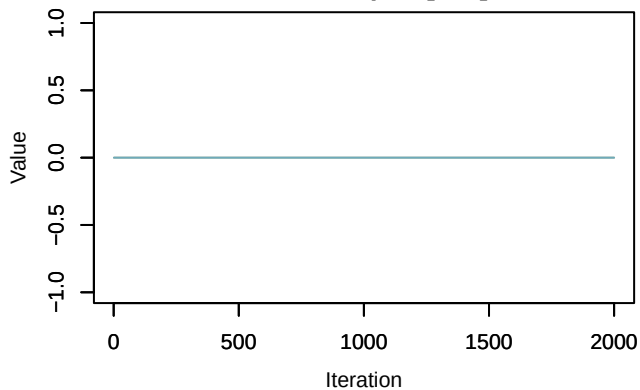
Trace – b_post[2, 3]
