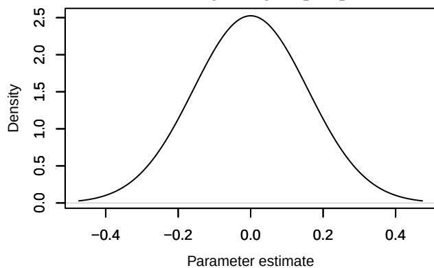
Density – b_post[2, 3]
