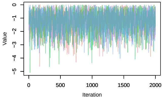
Trace – b_post[1, 1]
