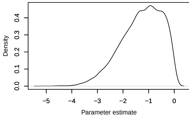
Density – b_post[1, 1]
