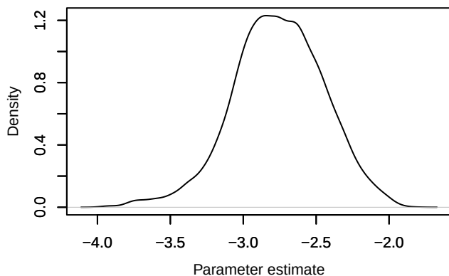
Density – b_postJ[1, 1]
