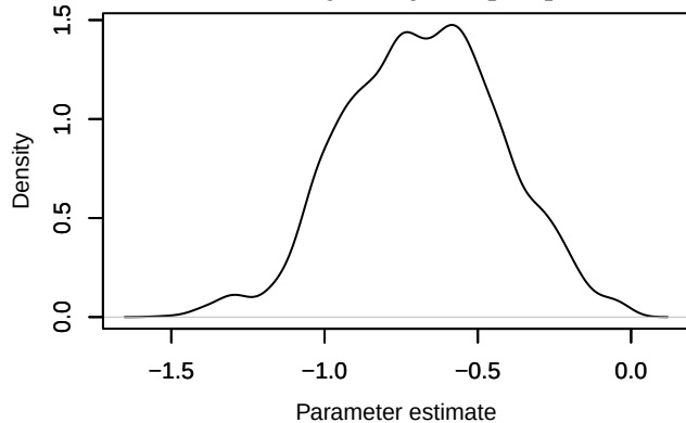
Density – b_postJ[2, 2]
