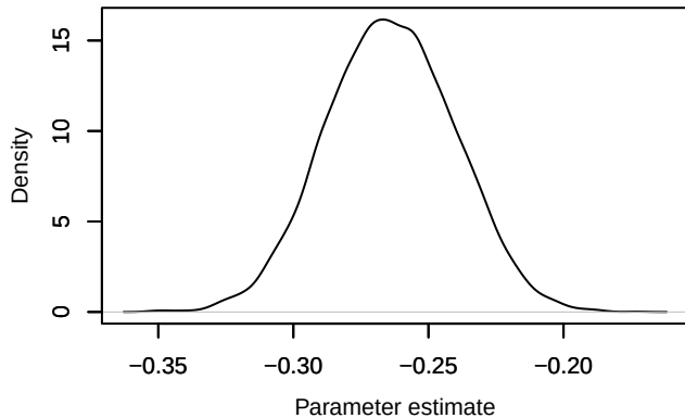
Density – lp[1, 3]
