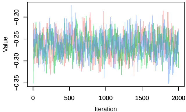
Trace – lp[1, 3]
