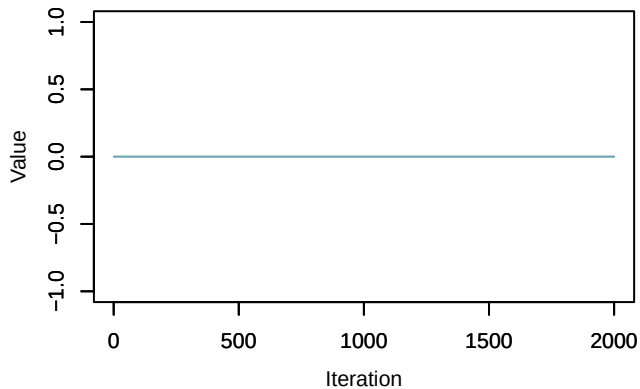
Trace – b_postJ[1, 3]
