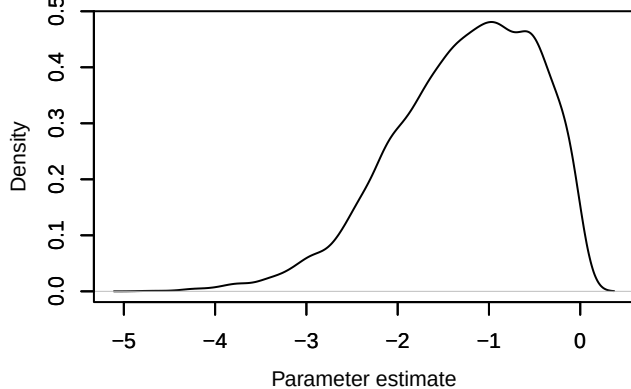
Density – b_postJ[2, 1]
