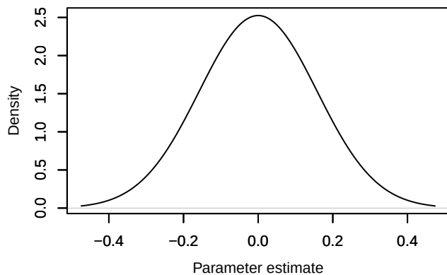
Density – b_postJ[1, 3]
