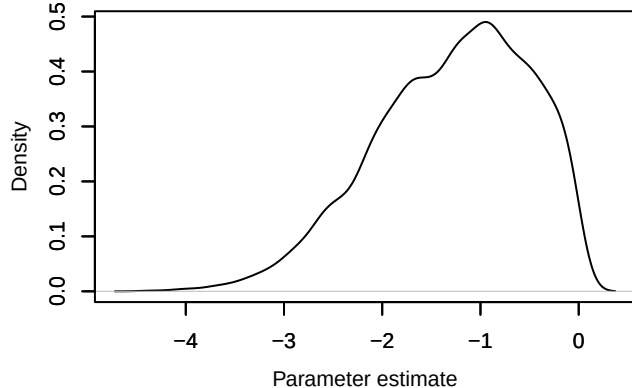
Density – b_postJ[2, 2]
