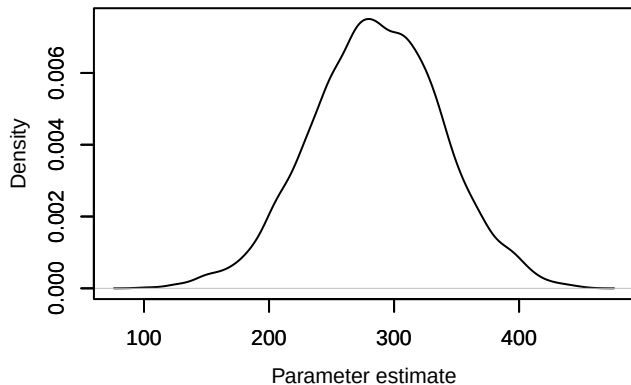
Density – U0[2, 3]
