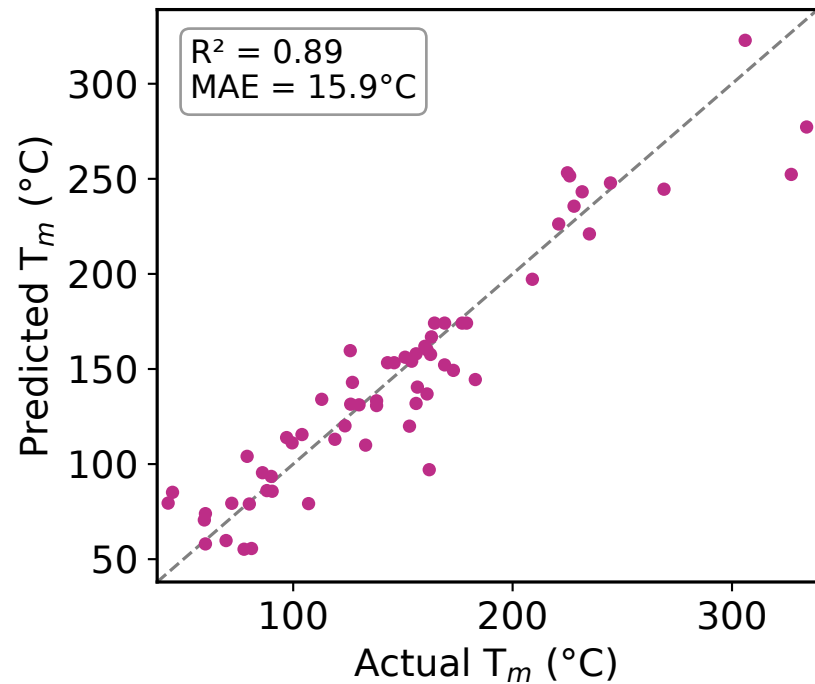
GATv2 (PBSG)
