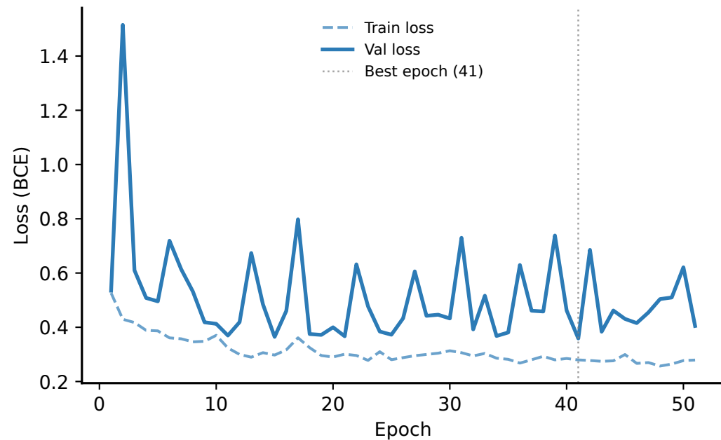
GINE (PBSG)
