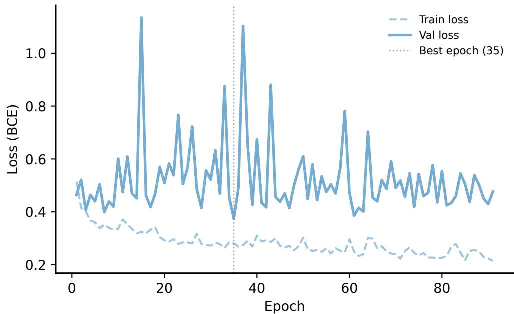
GATv2 (PBSG)
