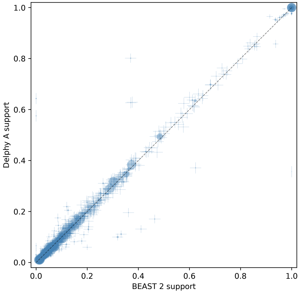
Clade posterior support (ESS: BEAST 2=480, Delphy A=490)
