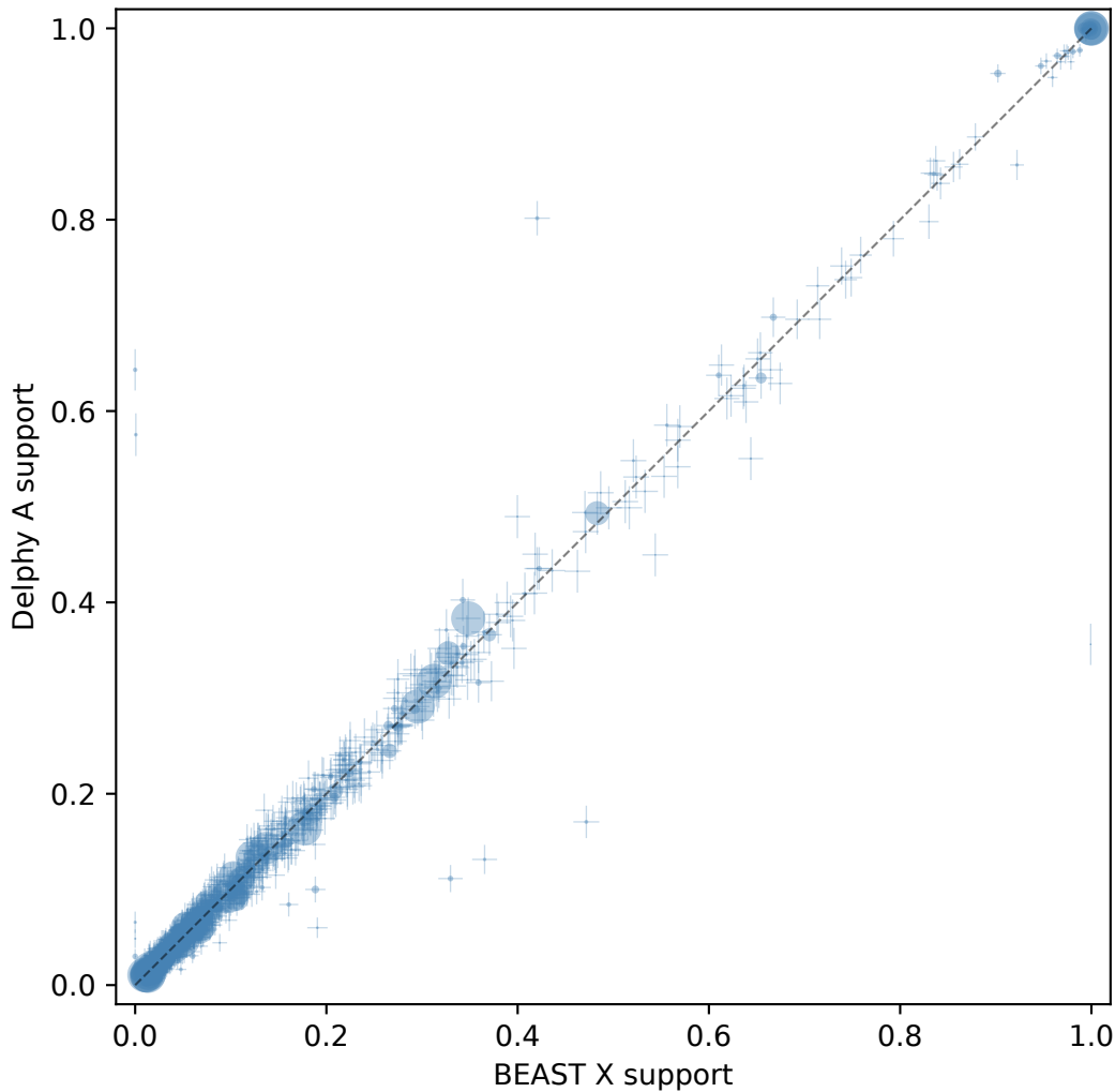
Clade posterior support (ESS: BEAST X=1359, Delphy A=490)
