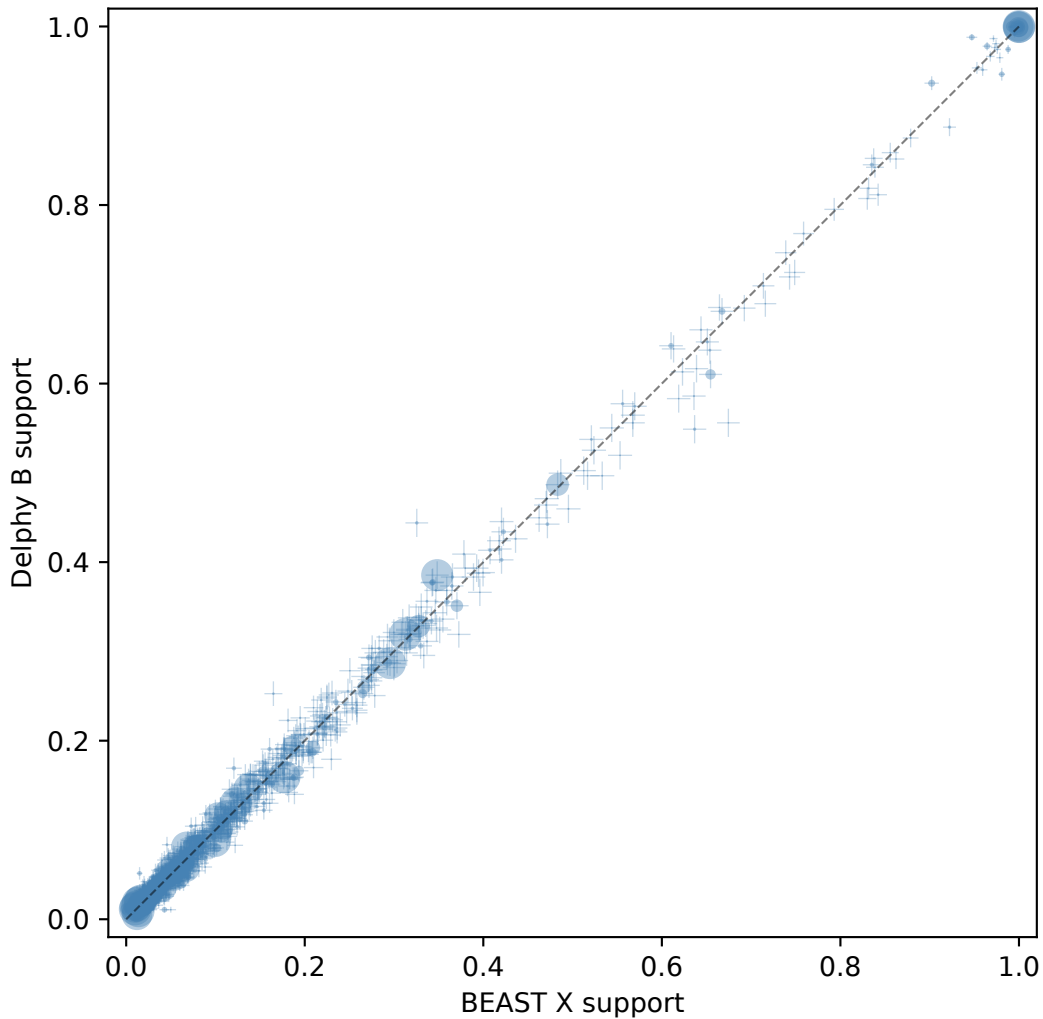
Clade posterior support (ESS: BEAST X=1359, Delphy B=988)
