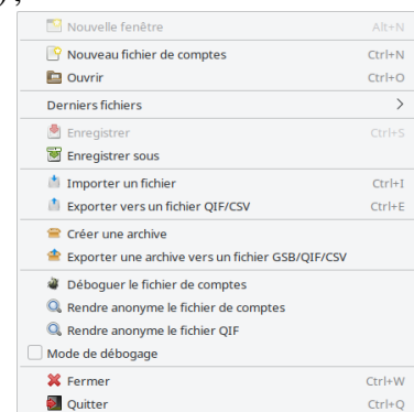
FIG. 4.5 Menu Fichier
