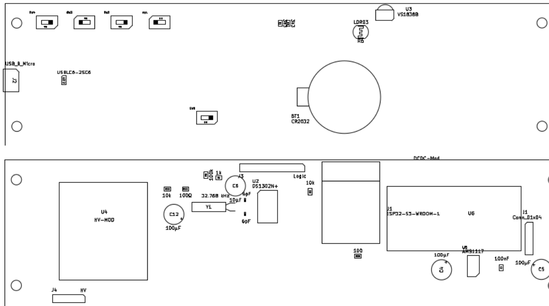
Abb. 2a – Logic Board Rev 2.1 PCB- Layout Oberseite
