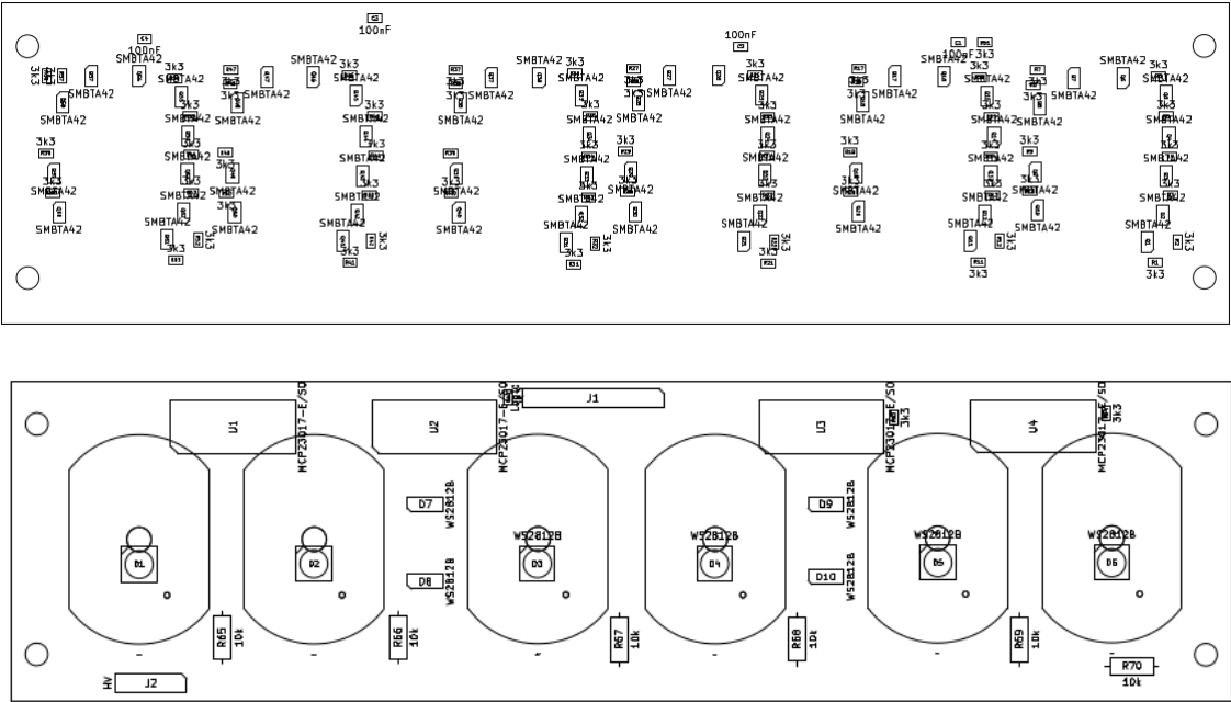
Abb. 4a – Nixie Display Board Rev 2.01 PCB- Layout Oberseite
