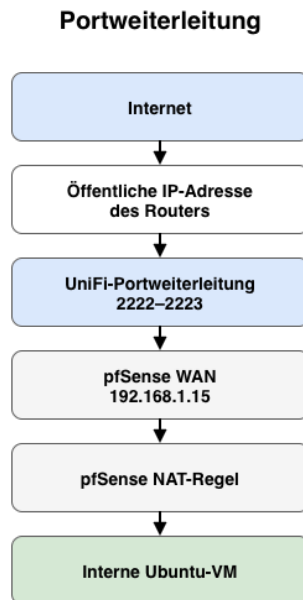
Figure 3: UniFi-Portweiterleitung
