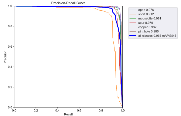
图 3 YOLOv5s 在官方测试集上的 PR 曲线 (mAP@0.5)。
