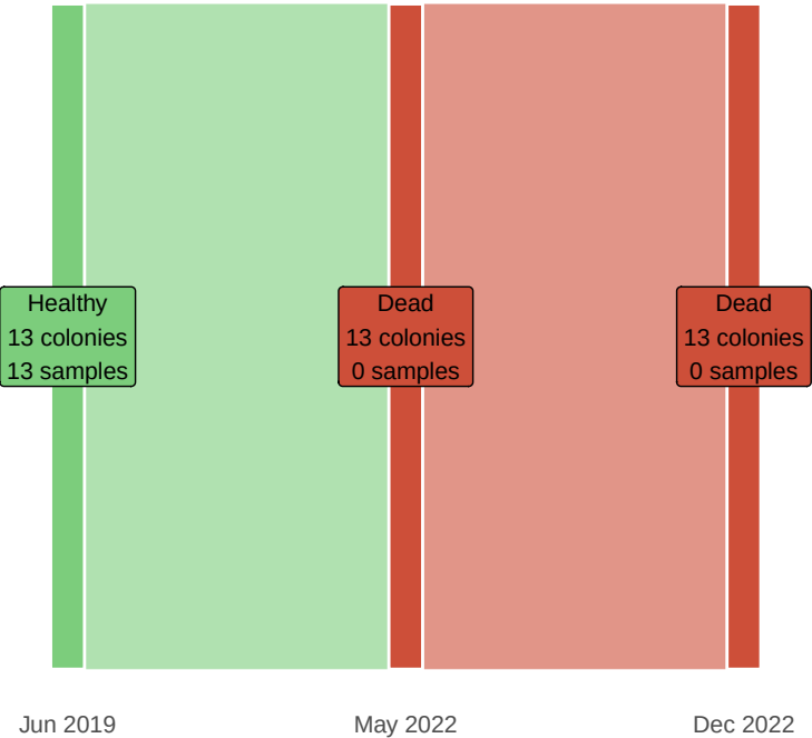
MMEA
