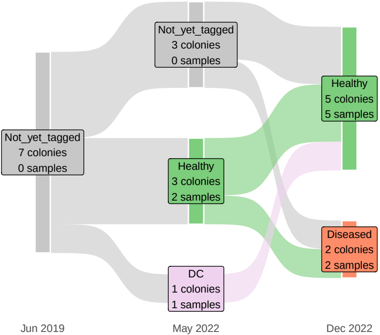
OFAV
