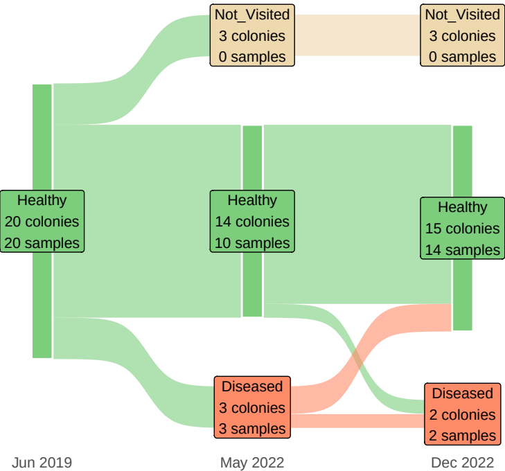
MCAV
