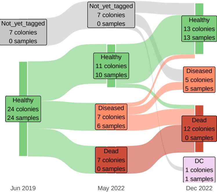
MMEA
