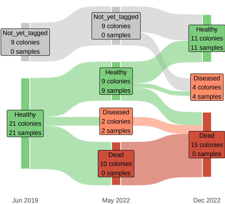
OANN
