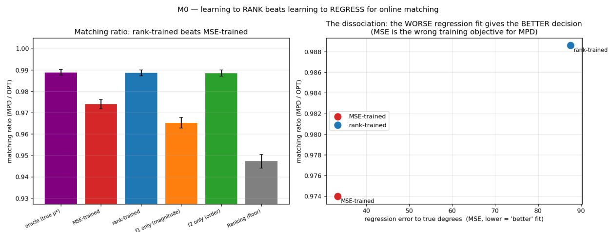
图 9: M0: 用发散特征时, rank 训练在匹配比值上击败回归 (左), 尽管其回归拟合更差 (右) ——这一解离表明回归对 MPD 是错误的训练目标。
