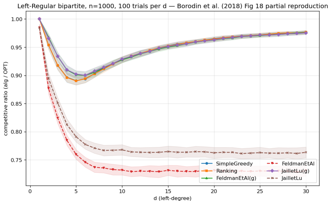
图 2: 随机左正则复现 (竞争比 vs 左度数 d ): 困难情形在 d = 5 、Greedy \approx Ranking、非贪婪退化。
