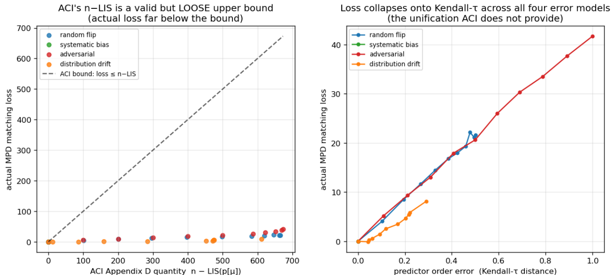
图 4: 顺序误差支配损失。(a) 实际 MPD 损失远低于 ACI 的 n - LIS 上界, 且 n - LIS 饱和。(b) 损失在四种误差模型上塌缩到 Kendall- \tau 顺序误差之上。
