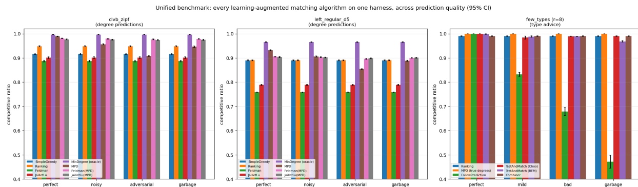
图 3: 统一基准: 竞争比 (均值, 95% 置信区间) 随预测质量的变化, 三个面板。裸跟随者 (对抗下的 MPD、FollowPrediction) 跌破免预测地板; 鲁棒算法则不会。
