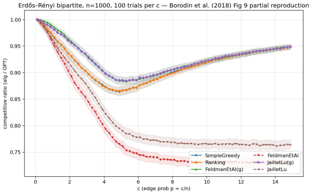
图 1: Erdős-Rényi 复现（竞争比 vs 边密度 c ）：特征性的 U 形、 c \approx 4.9 附近的贪婪最小值、以及非贪婪算法随 c 增大的退化。
