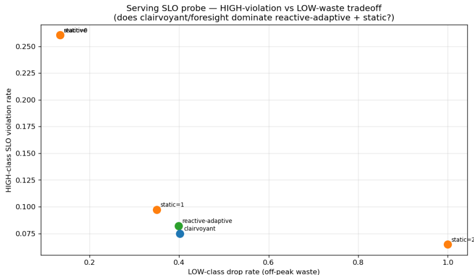
图 10: 服务 SLO 探针: 在突发负载下的紧 SLO/尾部目标上, 一个非预测策略 (静态余量或反应式自适应) 在几个百分点内匹配 clairvoyant 预言机——前瞻无济于事。
