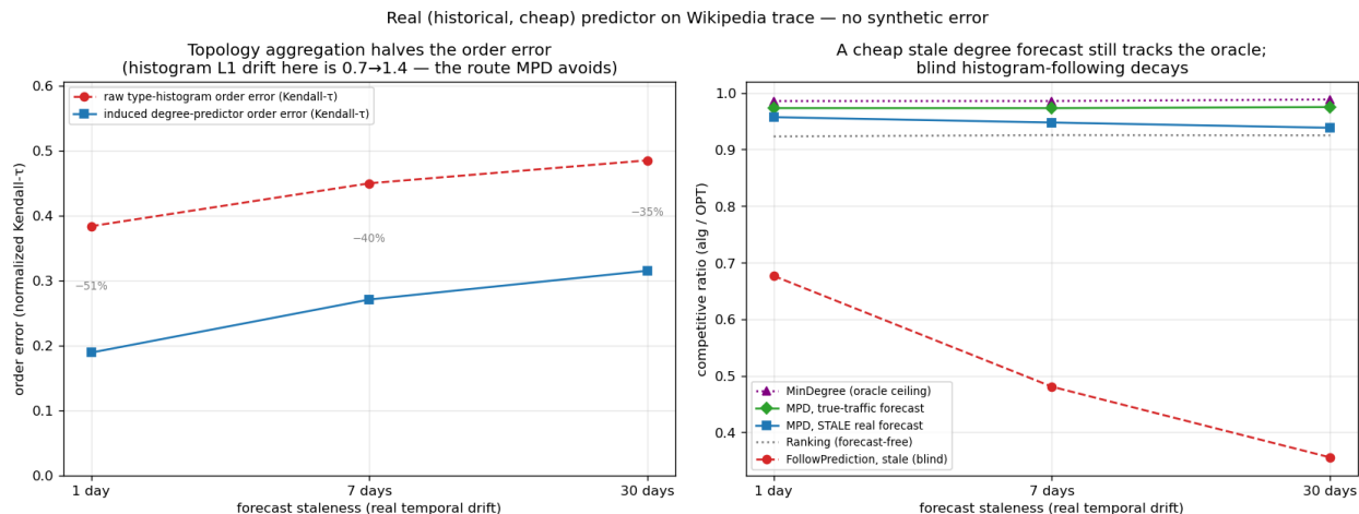
图 7: 一个真实、廉价的预测器 (Wikipedia trace)。(a) 拓扑聚合将诱导度数预测器的顺序误差降到原始直方图的一半。(b) 一个陈旧预测通过度数路线仍能跟住预言机, 而盲从直方图则衰减。
