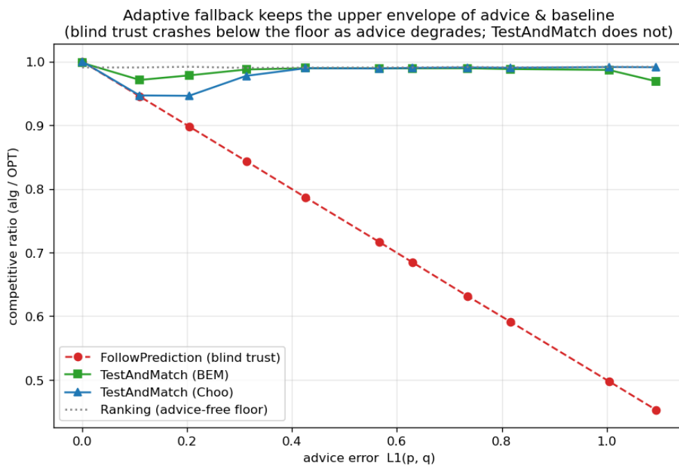
图 5: 鲁棒性包络。随建议误差 \ell_1(p, q) 增大, 盲从的 FollowPrediction 跌破免预测地板, 而 TestAndMatch (Choo/BEM) 稳在上包络。
