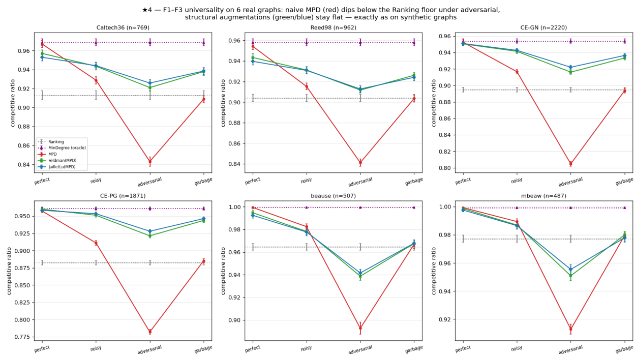
图 8: 六个真实图上的 F1-F3。裸 MPD (红) 在每个图上都在对抗预测下跌破 Ranking 地板; 结构式增强 (绿/蓝) 保持平坦——与合成图上一致。
