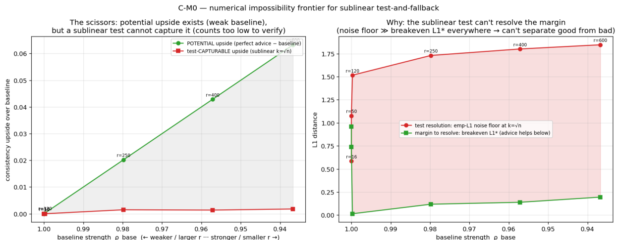
图 11: 不可能性的数值面(“剪刀”)。左: 随基线变弱, 潜在上升空间增长, 但亚线性检验能安全捕获的上升空间保持近零。右: 无论何处有上升空间, 检验的经验 \ell_1 分辨率都远高于盈亏平衡余量。
