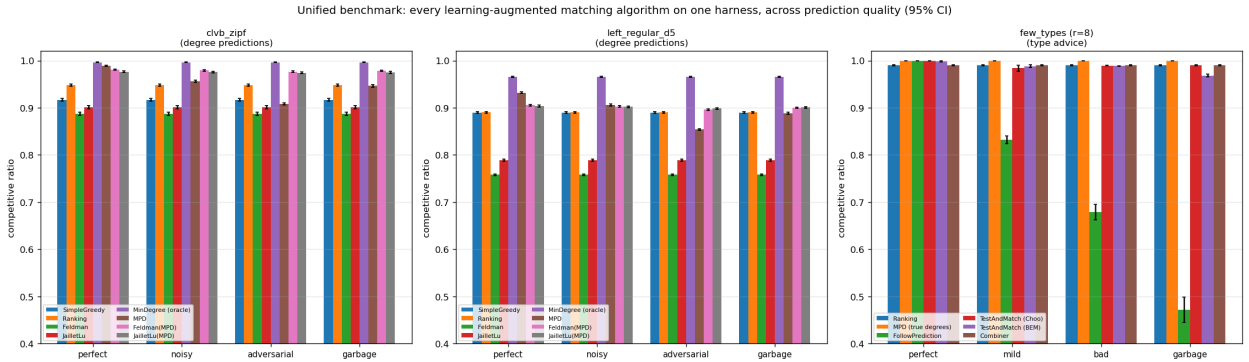
图 4.1: 统一基准：竞争比（均值，95% 置信区间）随预测质量的变化。裸跟随者跌破免预测地板；鲁棒算法则不会。
