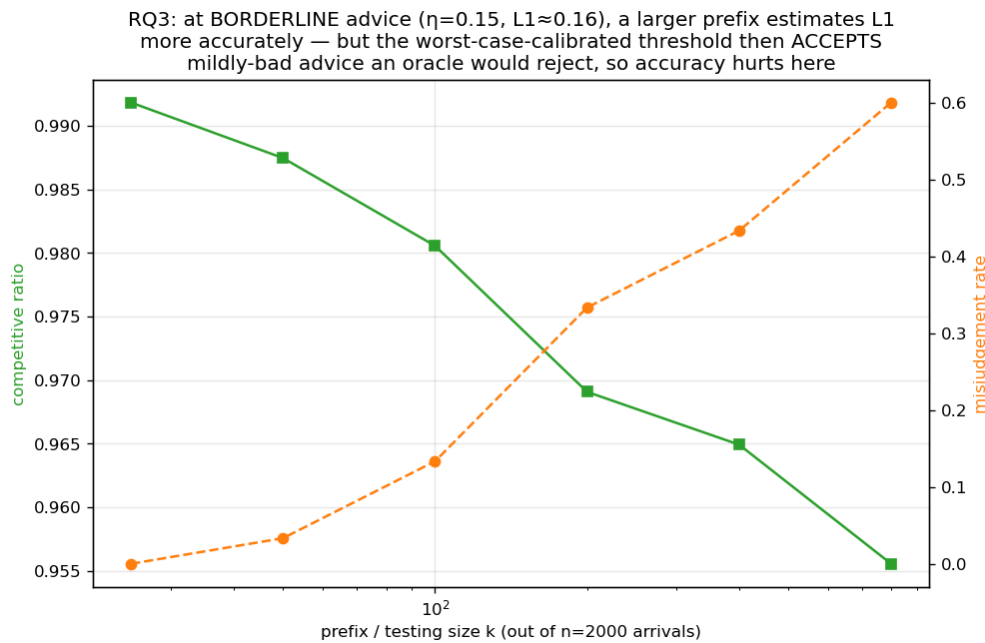
图 6.2: 边界建议下的检验代价: 一个更大、更准确的前缀检验反而做出更差的决策, 因为最坏情况校准的阈值在强基线输入上接受了轻度坏建议。
