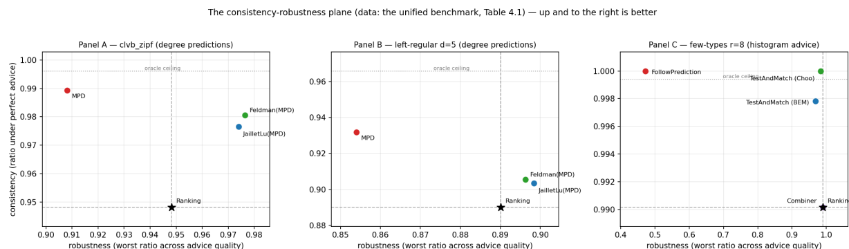
图 4.2: 一致性-鲁棒性平面, 每个算法一个点 (一致性 = 完美建议下的比值; 鲁棒性 = 各建议质量下的最差比值; 数据即表 4.1)。虚线为免预测地板, 点线为预言机天花板。朴素跟随者 (MPD、FollowPrediction) 用鲁棒性换一致性; 结构式增强两者都几乎不损失; TestAndMatch 最接近理想的右上角; combiner 钉在地板点上。
