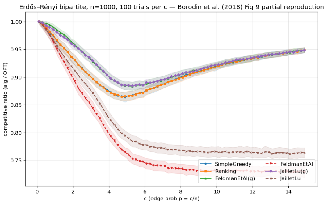
图 3.1: Erdős–Rényi 复现（竞争比 vs 边密度 c ）：特征性的 U 形、 c \approx 4.9 附近的贪婪最小值、以及非贪婪算法随 c 增大的退化。
