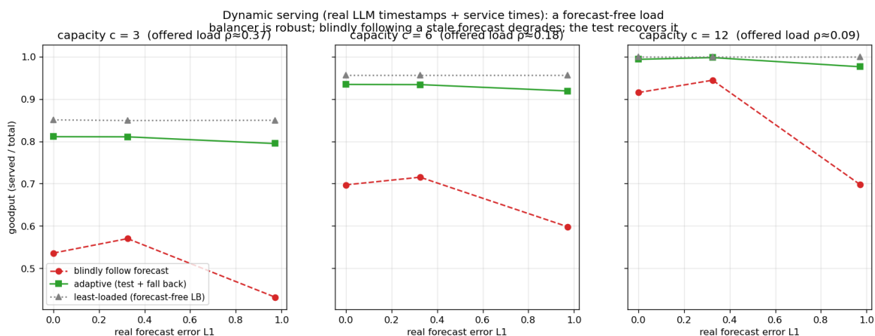
图 10.2: 预测 vs 实时负载 (真实 LLM 时间戳与服务时长): 免预测的最少负载均衡器在每个容量下都鲁棒, 而盲目跟随陈旧预测随其误差退化; 自适应检验挽回大部分差距。
