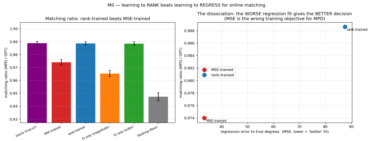
图 8.1: M0: 用发散特征时, rank 训练在匹配比值上击败回归 (左), 尽管其回归拟合更差 (右) —— 这一解离表明回归对 MPD 是错误的训练目标。
