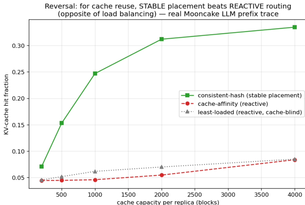
图 10.3: 缓存亲和反转（真实 Mooncake 前缀 trace）：对 KV 缓存复用， 稳定 的一致性哈希放置胜过反应式路由——与负载均衡情形相反——因为缓存局部性奖励持久性。
