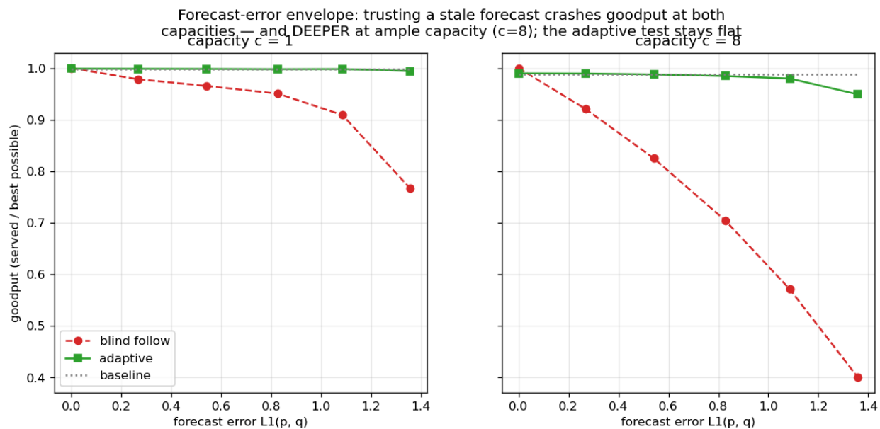
图 10.1: 容量作为鲁棒性: 随预测误差增大, 盲目跟随预测在两种容量下都使 goodput 崩塌——且在容量充裕 ( c = 8 ) 时摔得更深——而自适应检验则平贴在容量感知基线上。
