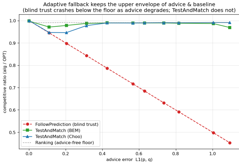
图 6.1: 鲁棒性包络。随建议误差 \ell_1(p, q) 增大, 盲从的 FollowPrediction 跌破免预测地板, 而 TestAndMatch (Choo/BEM) 稳在上包络。
