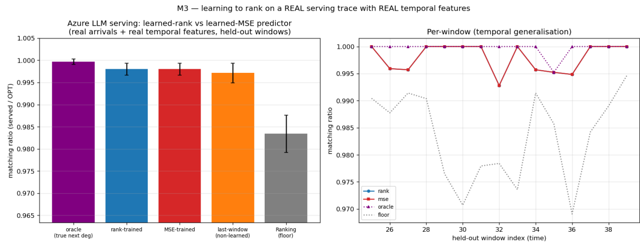
图 8.2: M3——真实 trace (Azure LLM) 上的决定性负结果: 在真实到达与真实时序特征下, rank 训练与 MSE 训练的预测器彼此不可区分、也与未学习的上窗口计数不可区分, 全都贴近预言机——驱动 rank 训练的人造顺序/幅度发散并不出现。
