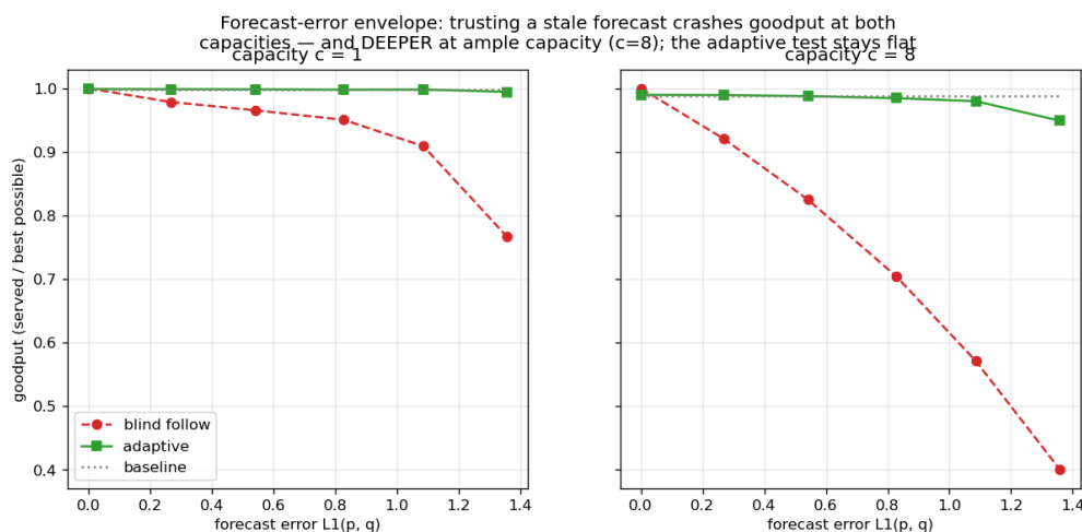
图 9.1: 容量作为鲁棒性：盲目跟随预测使 goodput 崩塌——容量充裕 ( c = 8 ) 时更深——而自适应检验保持平坦。
