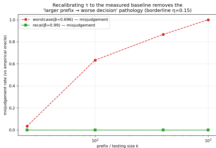
图 6.3: 重校准消除阈值病理: 误判率在每个前缀规模都保持为零, 而最坏情况阈值下攀向 1.0。
