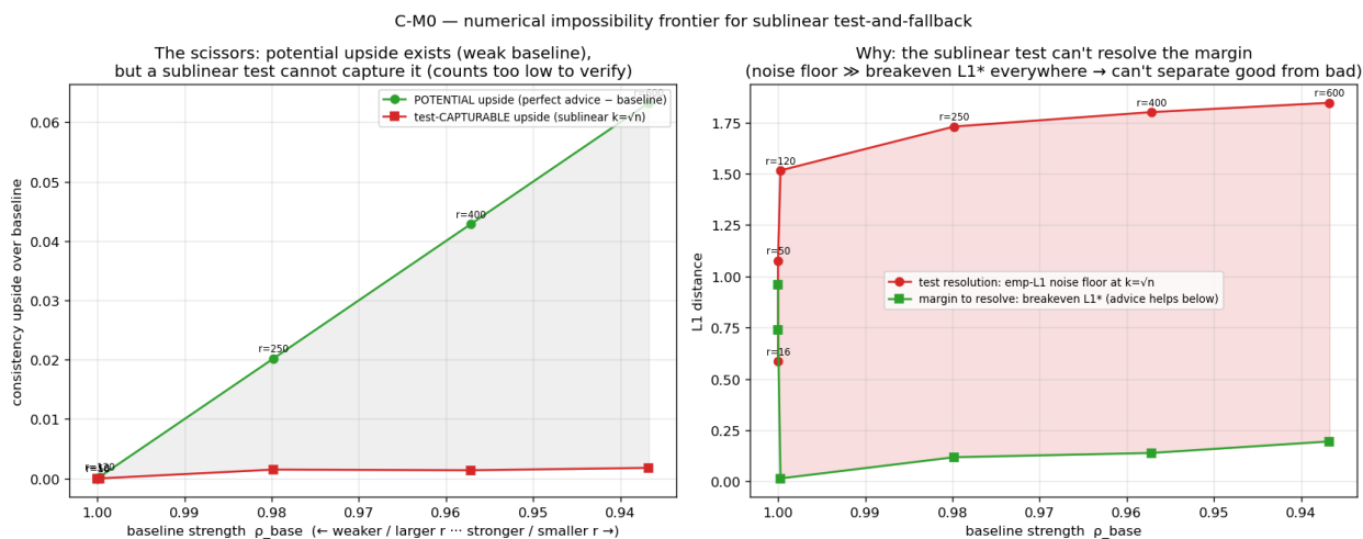
图 6.4: 检验之墙的境界图: 随基线变弱(左), 完美建议的潜在上升空间增大, 但亚线性检验能安全捕获的上升空间始终接近零——凡上升空间存在之处, 经验检验的分辨率都远高于盈亏平衡边际。
