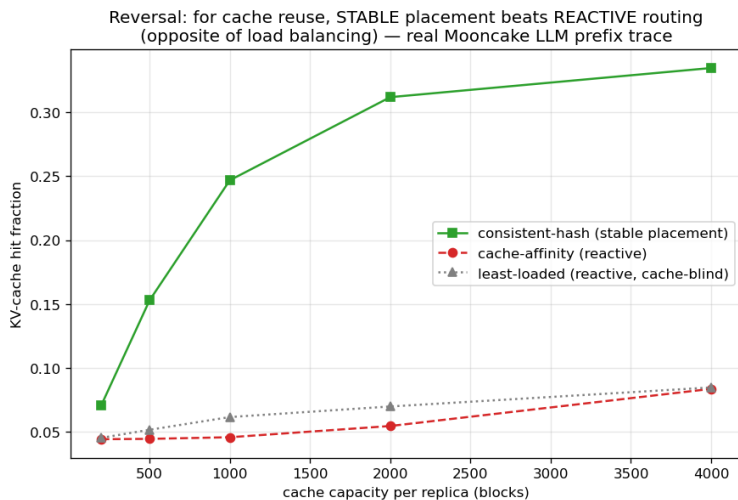
图 9.3: 缓存亲和反转 (Mooncake trace): 对 KV 缓存复用, 稳定放置胜过反应式路由。
