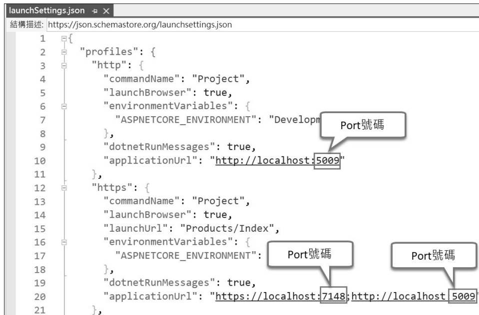
圖 2-20 修改專案的 SSL Port 號碼
