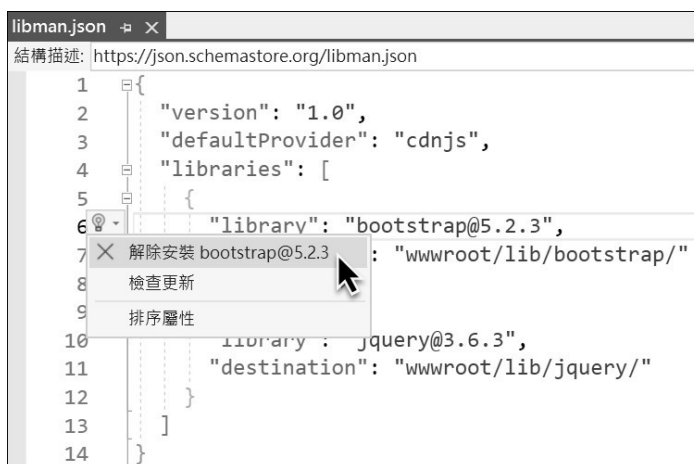
圖 2-28 用 LibMan 解除安裝函式庫
